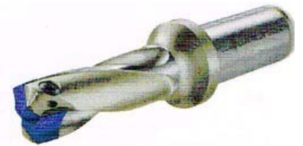
Schaft: zylindrisch mit Fläche Tige : cylindrique avec meplât
