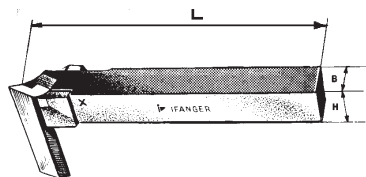
Typ E (links)
