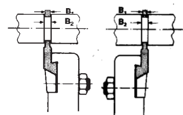
Halter Typ F Messer Typ FSE (rechts) à droite/right
