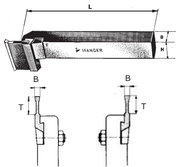
Typ F (rechts)
