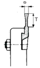
Typ G (links)
