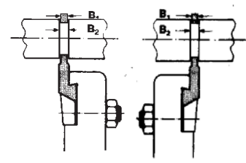
Halter Typ F Messer Typ FSE (rechts) à droite/right
