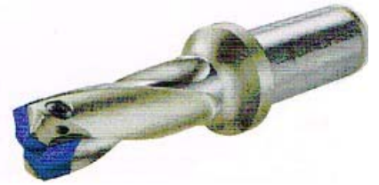
Schaft: zylindrisch mit Fläche Tige : cylindrique avec meplât
